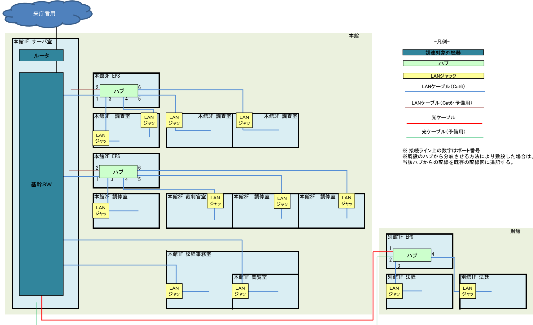
配線図(例)
