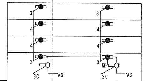
S宿舎1棟 系統図
