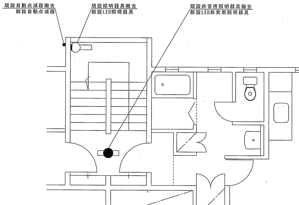
S宿舎2棟 平面図
