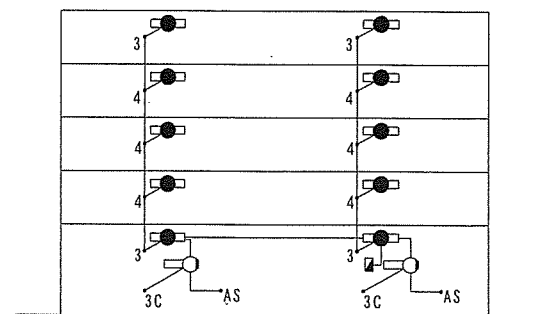
T宿舎 系統図
