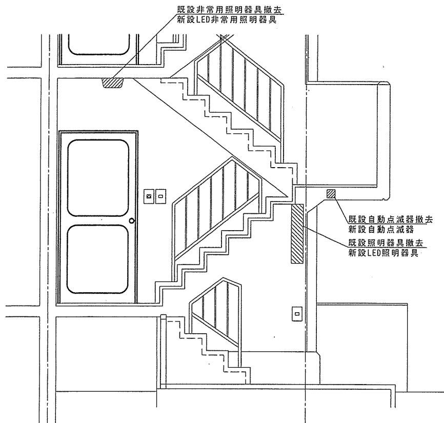
S宿舎2棟 階段部立面図
