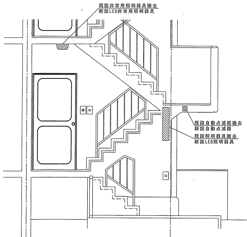
S宿舎1棟 階段部立面図
