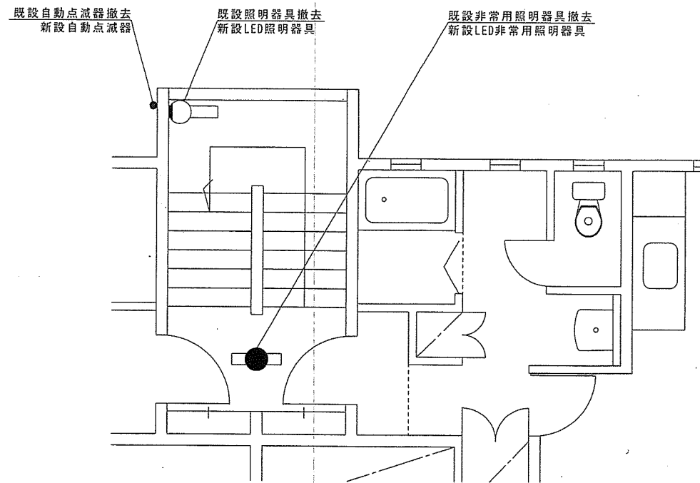
S宿舎1棟 平面図
