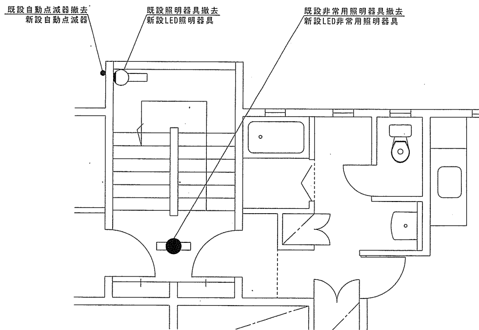
T宿舎 平面図
