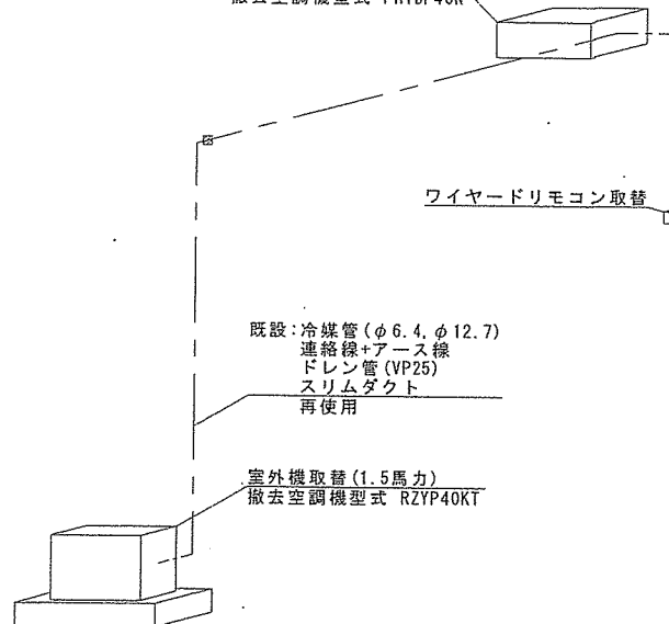
配管系統図
