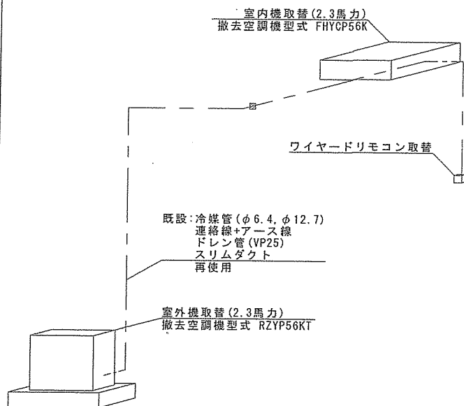
配管系統図
