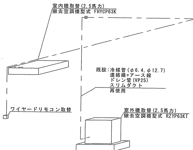
配管系統図
