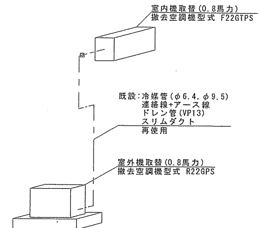
配管系統図
