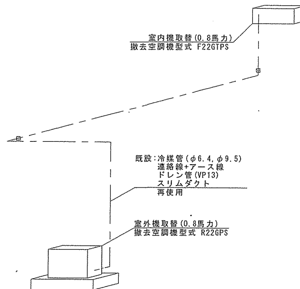
配管系統図
