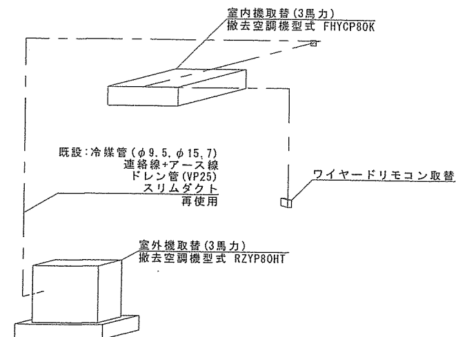
配管系統図
