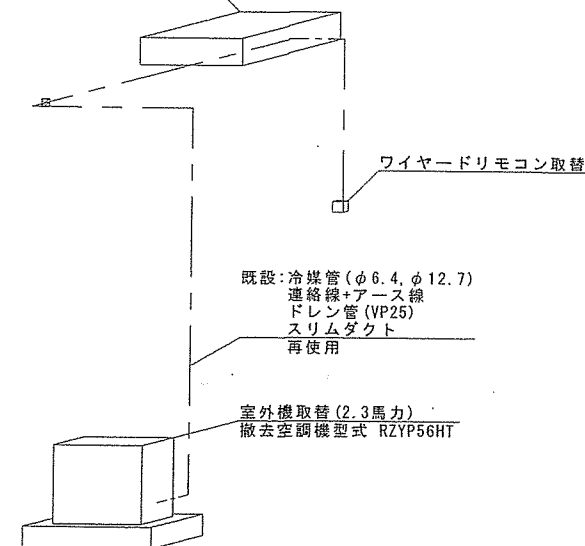
配管系統図
