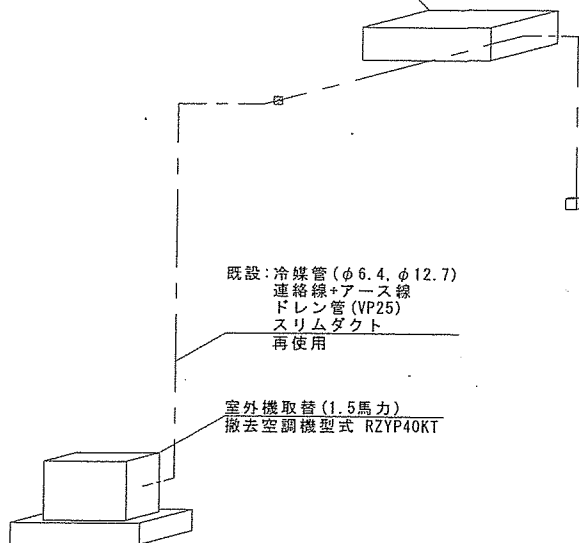
配管系統図
