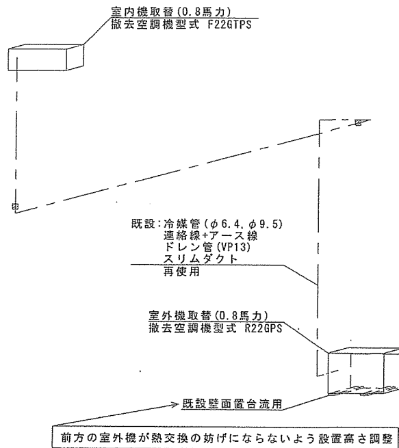
配管系統図
