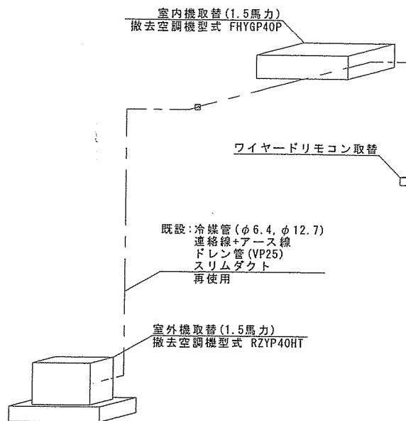
配管系統図
