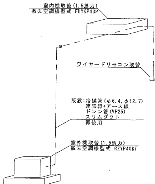
配管系統図
