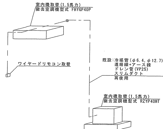
配管系統図
