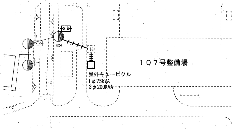
更新高圧ケーブル系統図
