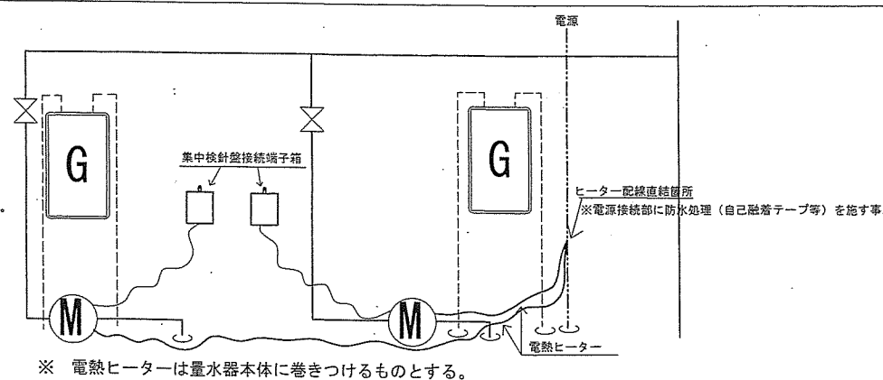
2～4Fパイプシャフト内配管系統図 S=1/S
