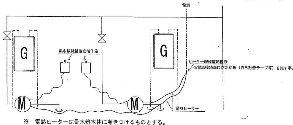
1Fパイプシャフト内配管系統図 S=1/S
