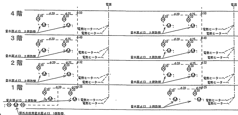
給水管系統図 S=1/X
