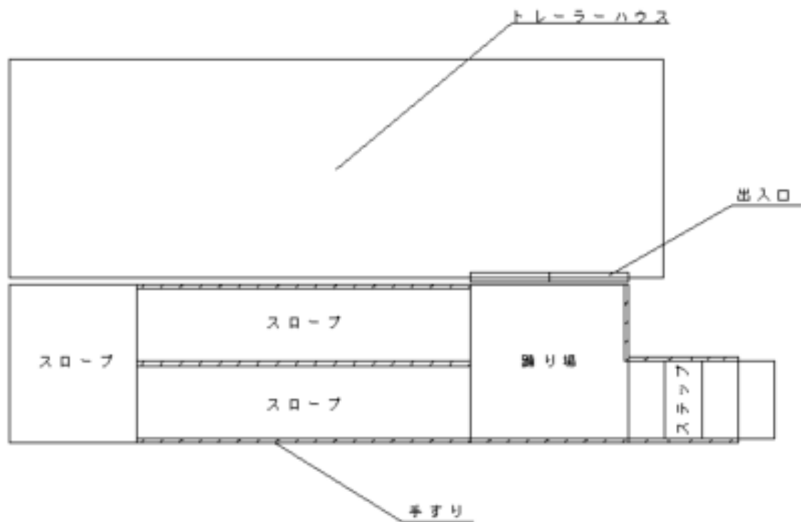
設置品基準図
